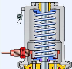
Индикатор подъема в кожухе J38: Переходник кожуха для клапана размером 1" J93: Индикатор подъема
