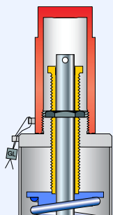
Герметичный рычаг H4 H4
