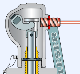
Индикатор подъема H4 Размер клапана от 1 1/2" до 3" J39: Переходник H4 J93: Индикатор подъема
